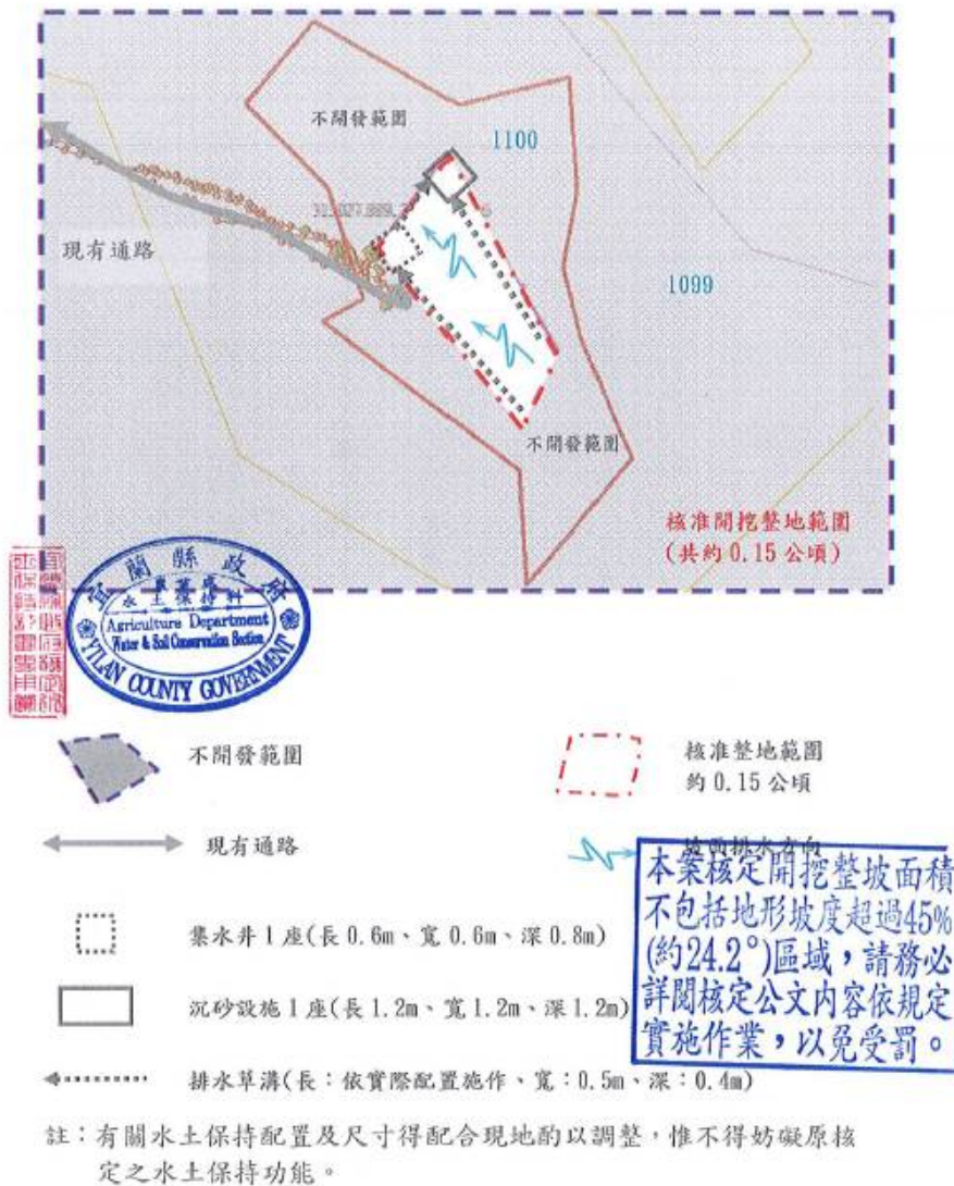
三星鄉天山段 1100 地號簡易水土保持設施平面配置示意圖
