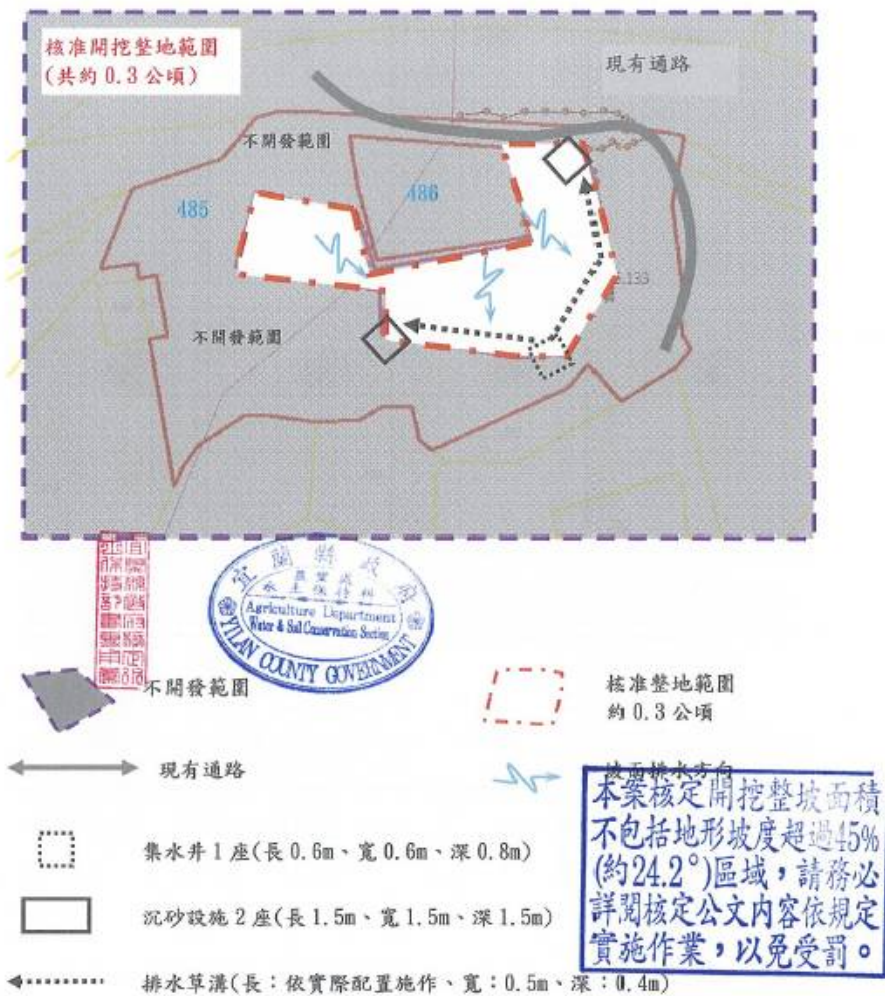
三星鄉柑仔坑段 485 地號簡易水土保持設施平面配置示意圖
