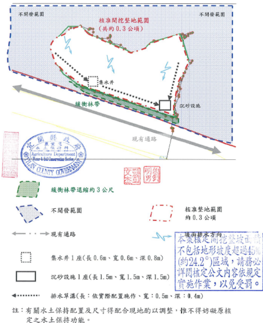
三星鄉天山段 594 地號簡易水土保持設施平面配置示意圖
