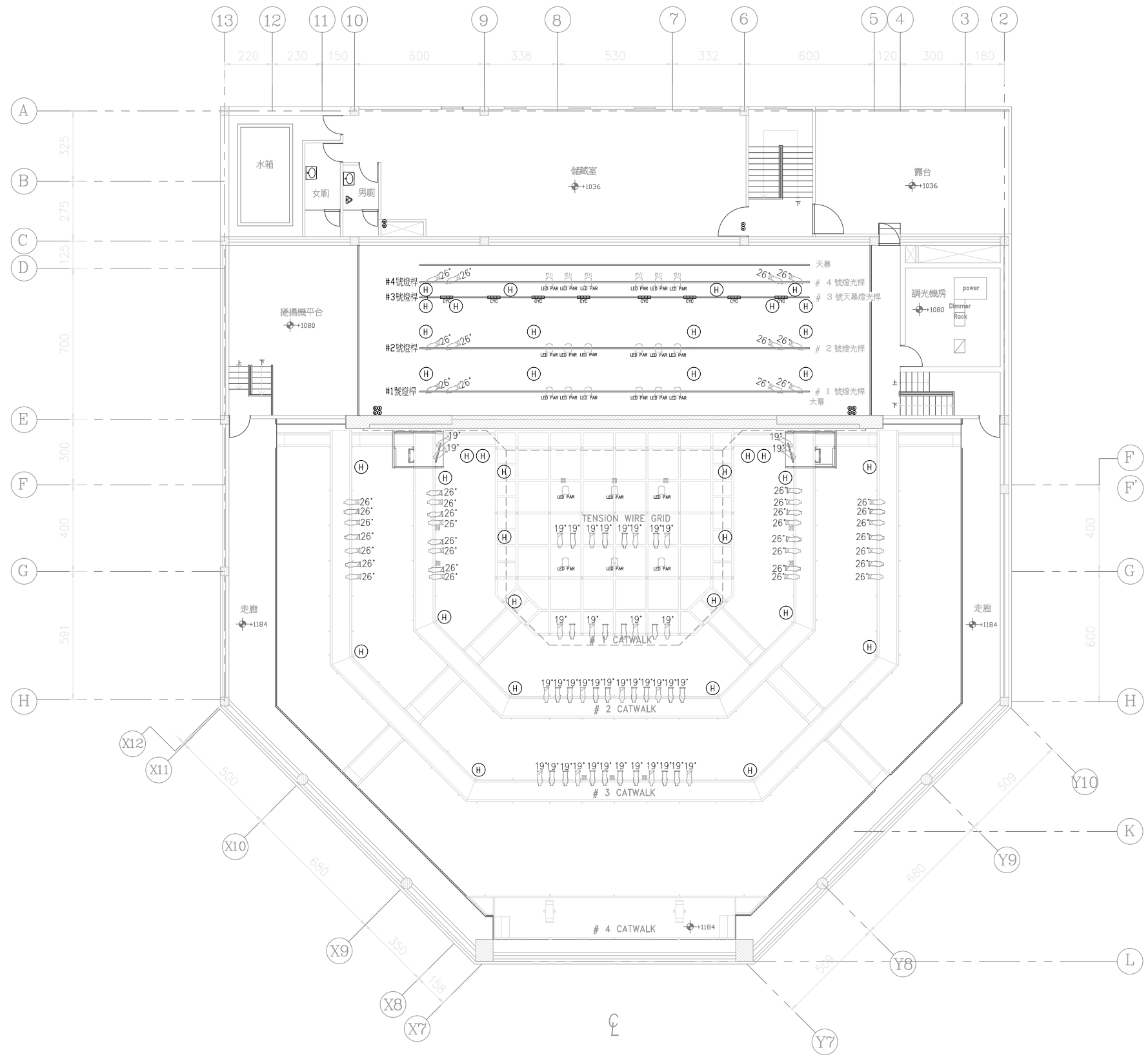
宜蘭縣政府文化局演藝廳燈具配置圖
