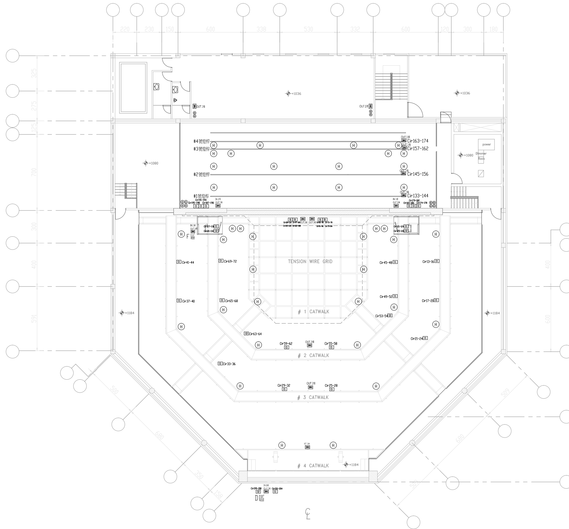
宜蘭縣政府文化局演藝廳燈光迴路配置圖
