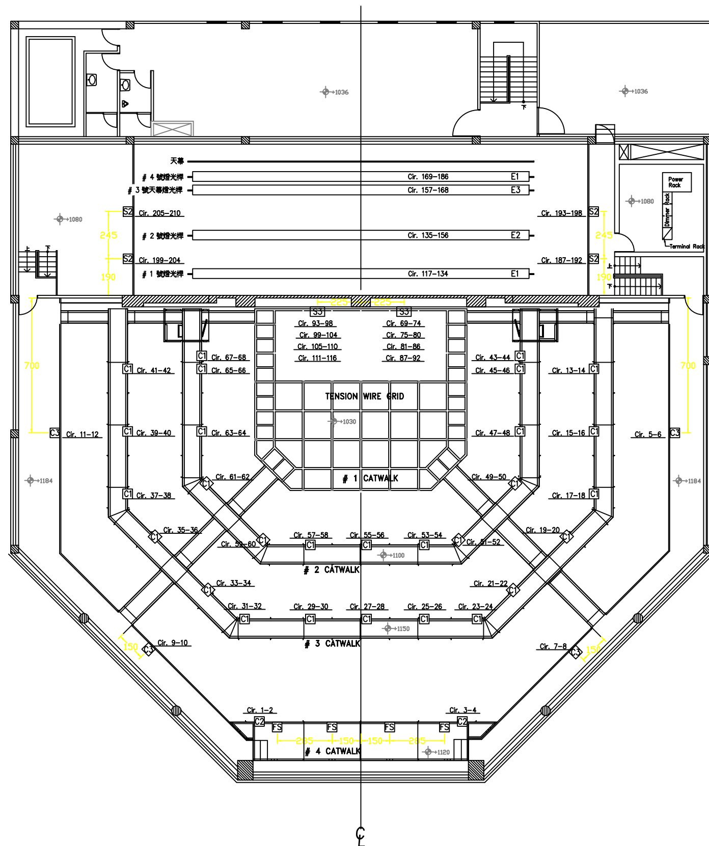
宜蘭縣政府文化局演藝廳燈光迴路圖
