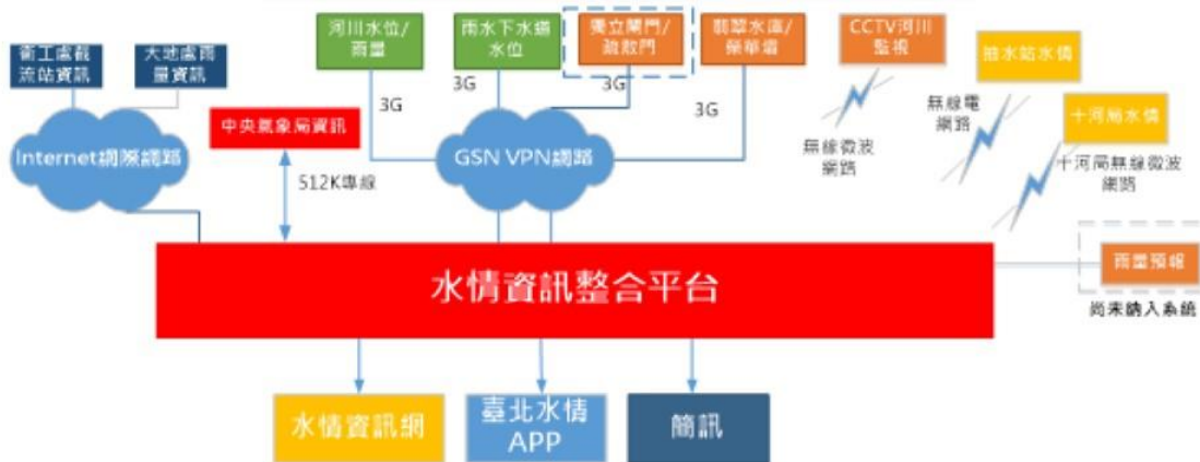
本市水情資訊接收管道架構圖
