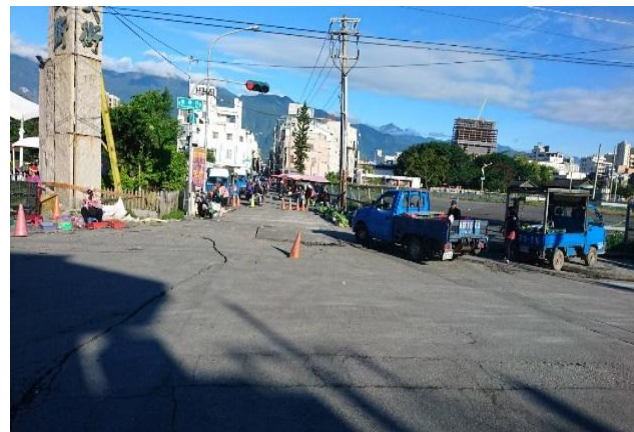
重慶路/博愛街路面裂縫、擠壓隆起
