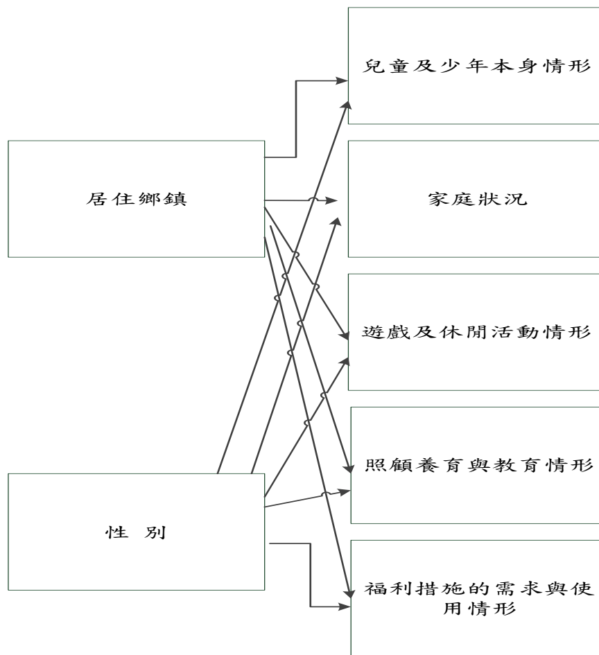
圖 1 研究架構圖
